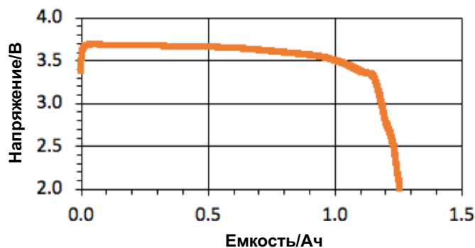
График разряда током 50 мА при температуре 180°C
